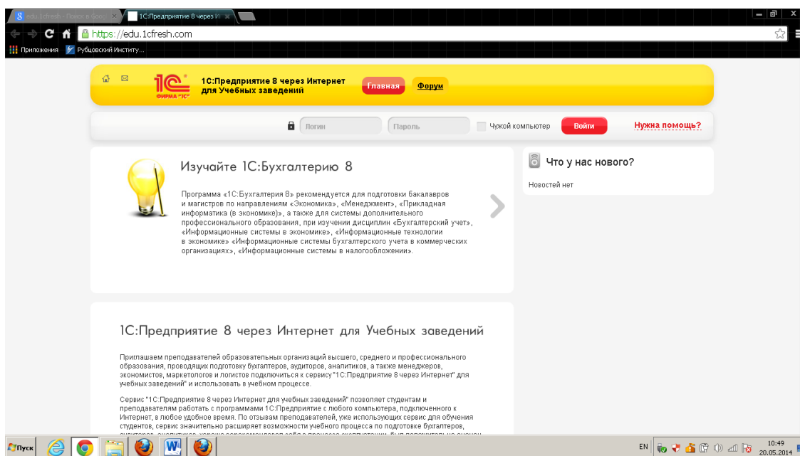
Рисунок 1 – Окно авторизации
